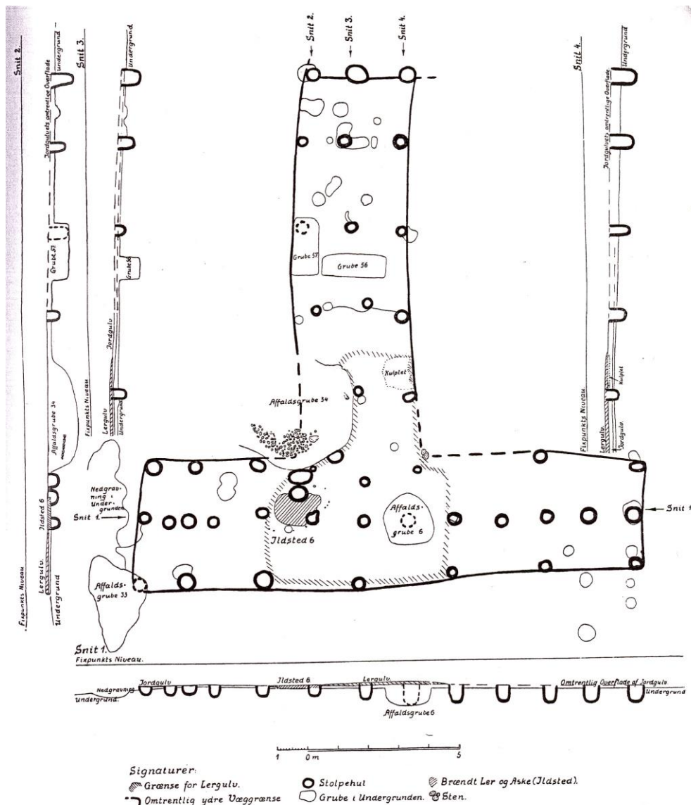
Plan af middelalderens Pebringegård med to sammenbyggede længer, hus II i Ø.-V., hus III i N.-S. Husene havde bulvægge, og taget blev båret af svære »midtsuler«. I midten af hus II var der opholdsstue med åbent ildsted, i vest formentlig et kammer eller herberg og i østenden (til højre) stald. Hus III's sydende hørte til beboelsen, medens resten vel var lade.
